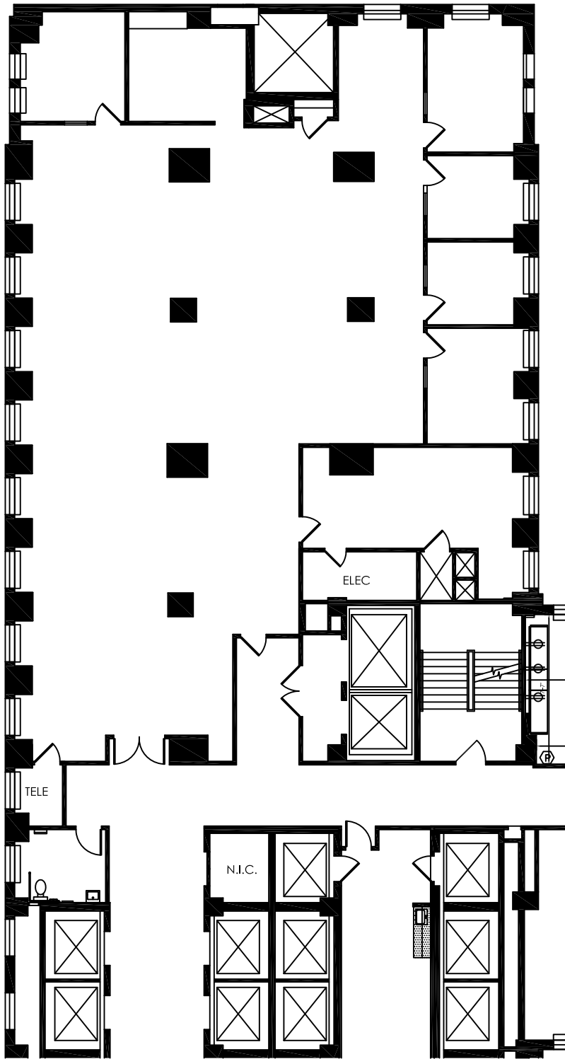
1 PLAN SCALE: 1/16" = 1'-0"
